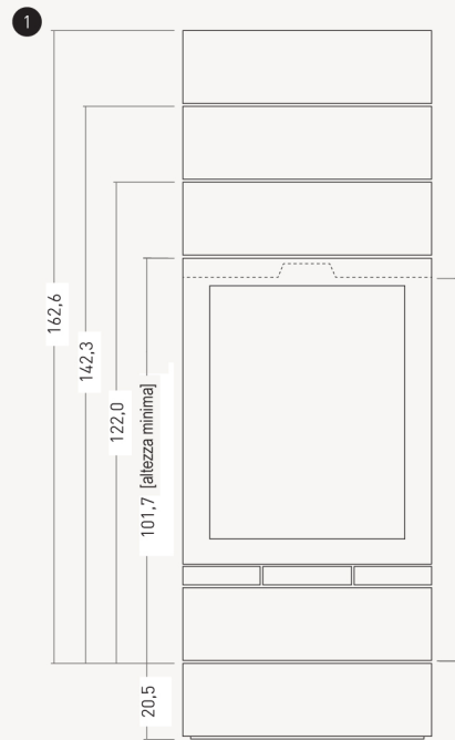
vista frontale
