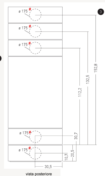
vista posteriore
