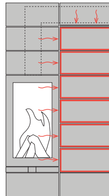
Optik-Boxen mit Strahlschutzsätzen
