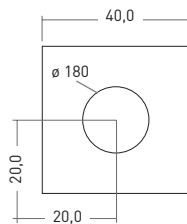
Rauchrohrabgang (oben)
