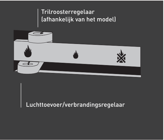
AFB. 3.2 Schuifstelsysteem, variant 1
