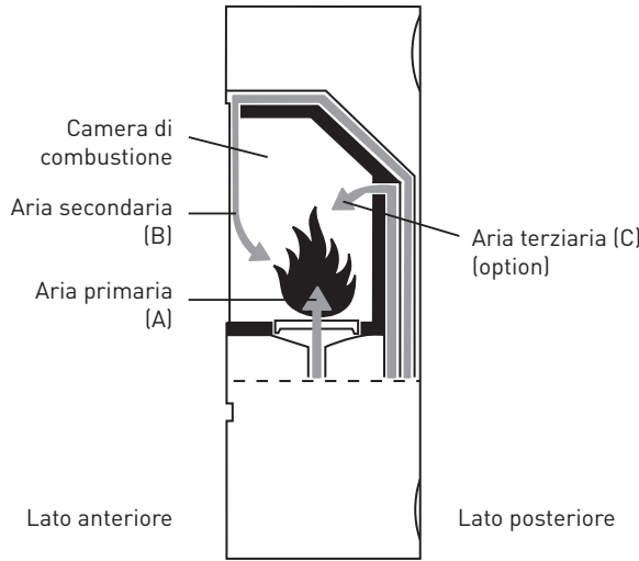
FIG. 3.1 Aria comburente, sezione della camera di combustione
