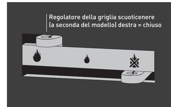
FIG. 4.13 Sistema a scorrimento, versione 1
